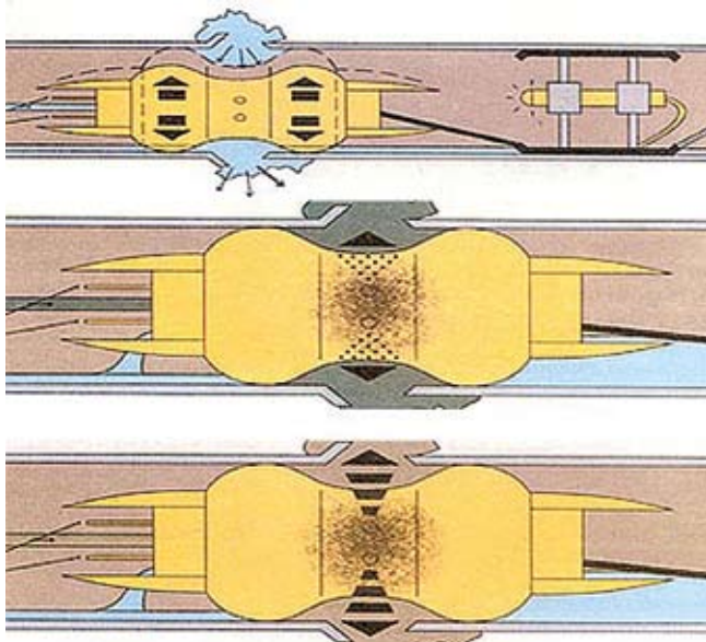
Rys. 3. Technologia naprawy miejscowej uszkodzonego rurociągu za pomocą pakera iniekcyjnego [20]
