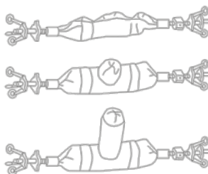
Rys. 29. Montaż kształtki kapeluszowej w przykanaliku [20]
