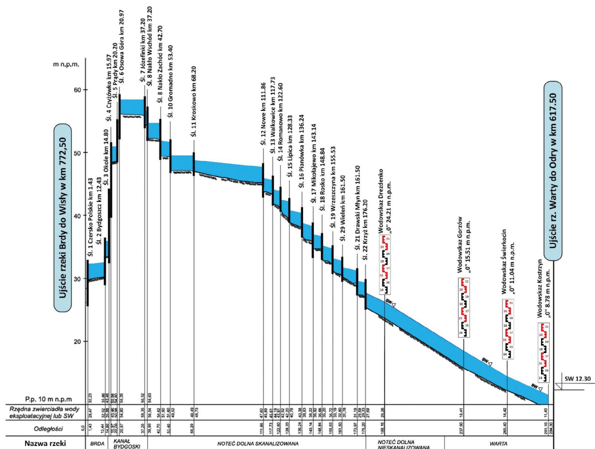
Rys. 3. Profil podłużny drogi wodnej Wisła-Odra
