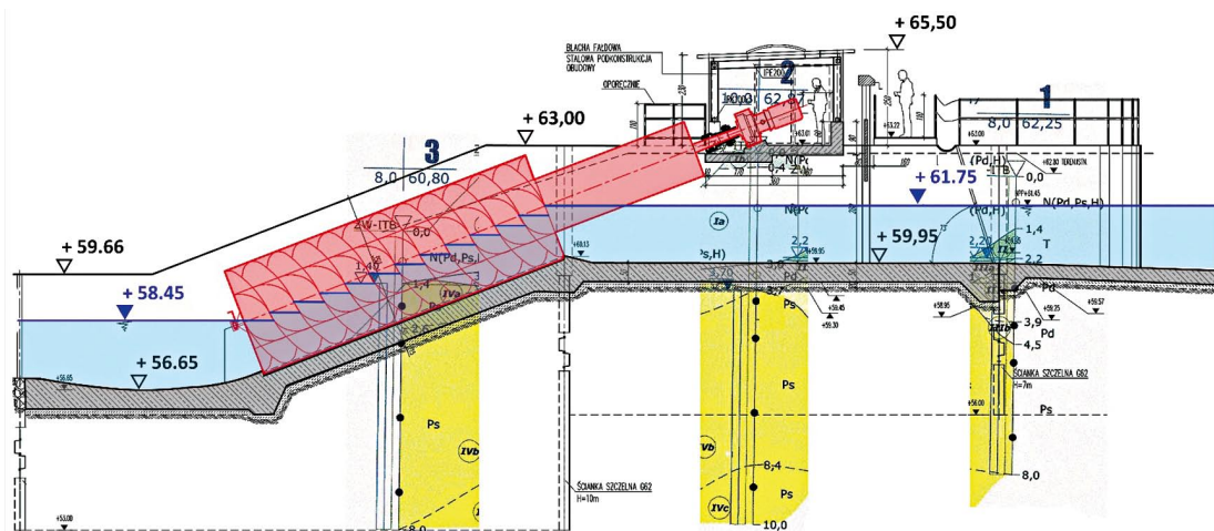
Rys. 9. Mała Elektrownia Wodna Lisi Ogon. Przekrój podłużny. Turbina Archimedes [6]
