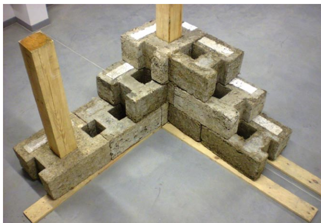
Rys. 3. Przykładowy narożnik ściany wykonany z wytworzonych pustaków z ekologicznym wypełniaczem organicznym
